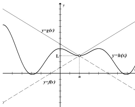
Ilustración del Teorema del encajonamiento
